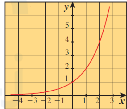
نمو أسي
