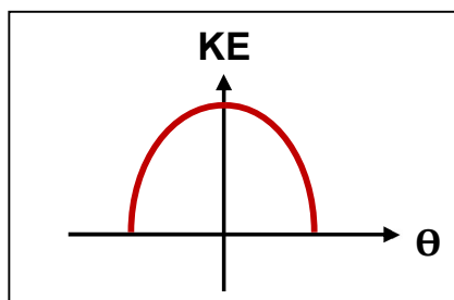
طاقة الحركة وزاوية البندول
