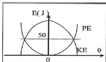
طاقة الوضع وطاقة الحركة للبندول
