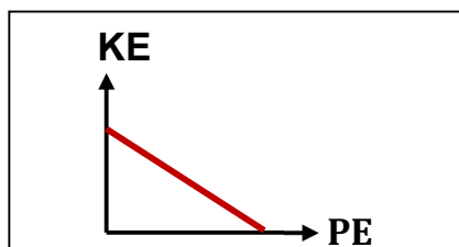
طاقة الوضع وطاقة الحركة للبندول
