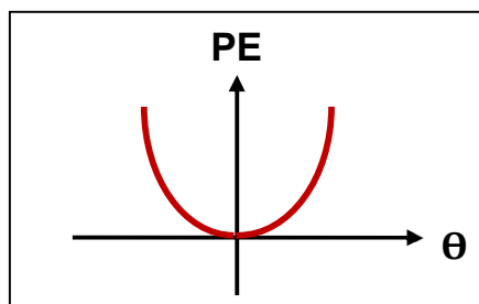
طاقة الوضع وزاوية البندول
