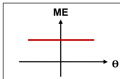
الطاقة الميكانيكية وزاوية البندول
