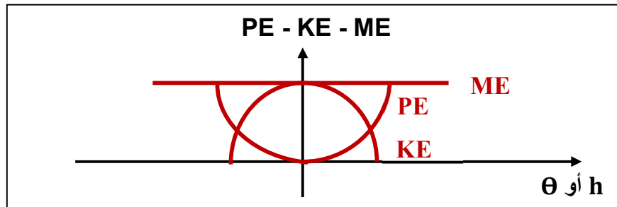
طاقة الوضع وزاوية البندول
