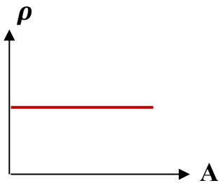
المقاومة النوعية للمادة ومساحة مقطع السلك
