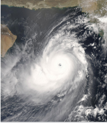
شكل ( ٥ ) صورة إعصار جونو ملتقطة من الأقمار الصناعية
