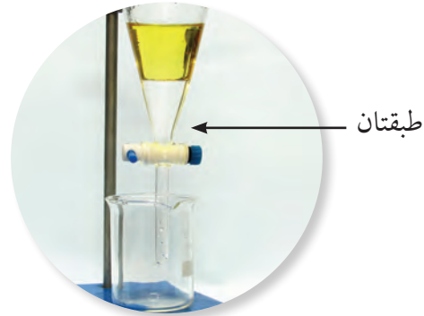
الشكل (١٨) قمع الفصل
