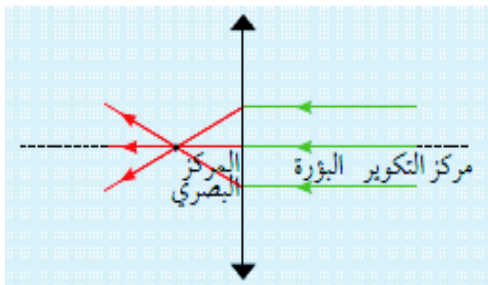
بؤرة العدسة المحدبة حقيقية
