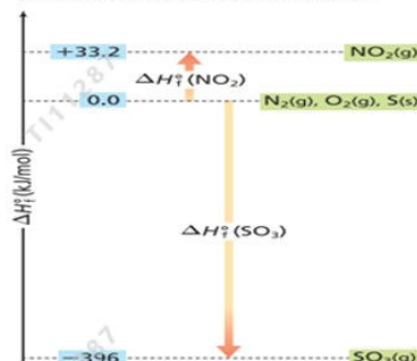
حرارة التكوين القياسية Standard Heat of formation
