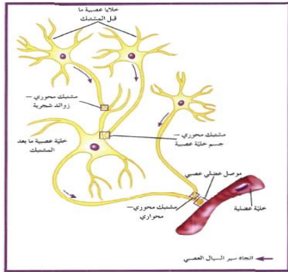
شكل (18) مواقع المشتبكات العصبية واتجاه انتقال الرسائل العصبية بين الخلايا.
