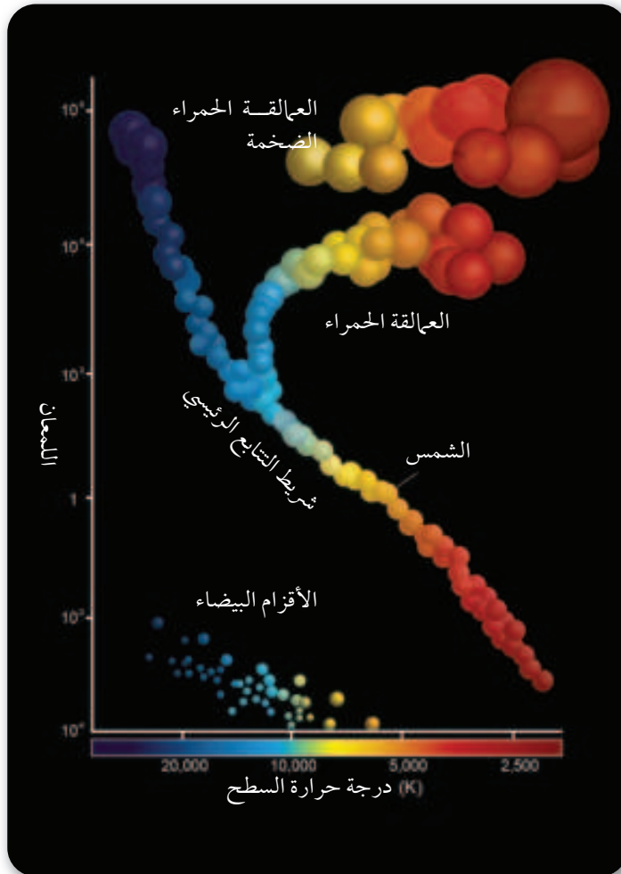
الشكل 12-1 H-R المخطط الذي يوضح مواضع النجوم بحسب درجة الحرارة واللمعان.
