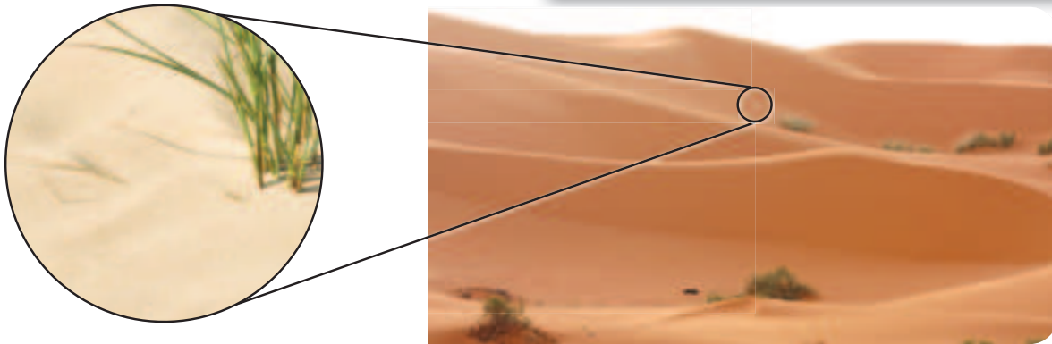
الشكل 18-4 تشكّلت هذه الكثبان من الرمل الذي عصف به الريح، فنقلته وأعادته ترسيبه. لاحظ أن حبيبات الرمل متساوية في الحجم تقريباً.
