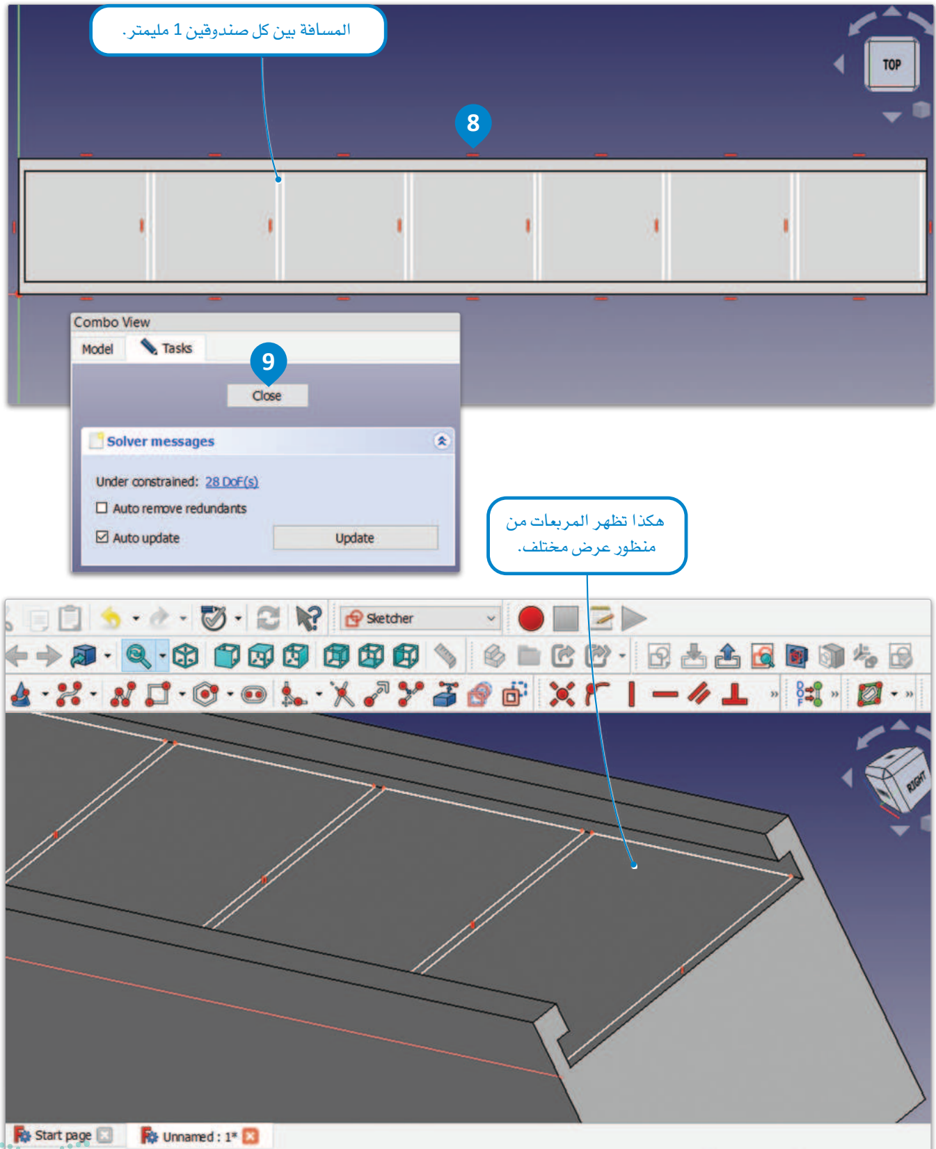
شكل 3.49: إنشاء سبعة مربعات
