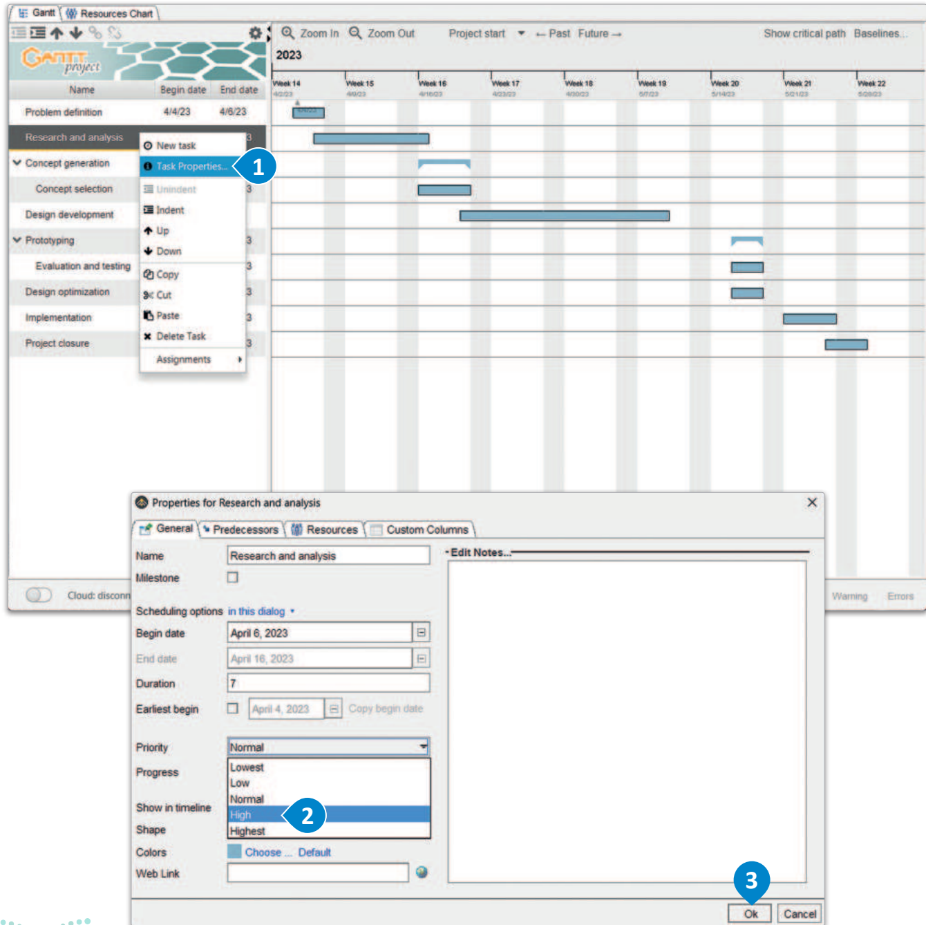
شكل 1.29: تغيير أولوية المهمة
