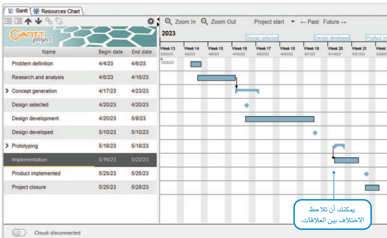
شكل 1.34: إضافة العلاقات بين المهام
