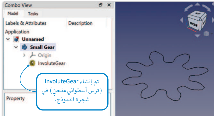
شكل 2.45: إضافة ترس أسطواناني منحني
