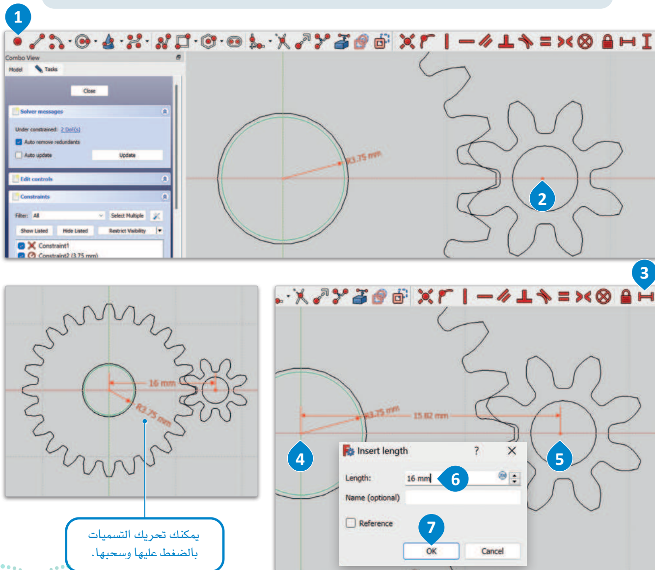
شكل 2.64: إنشاء مركز الدائرة الصغيرة
