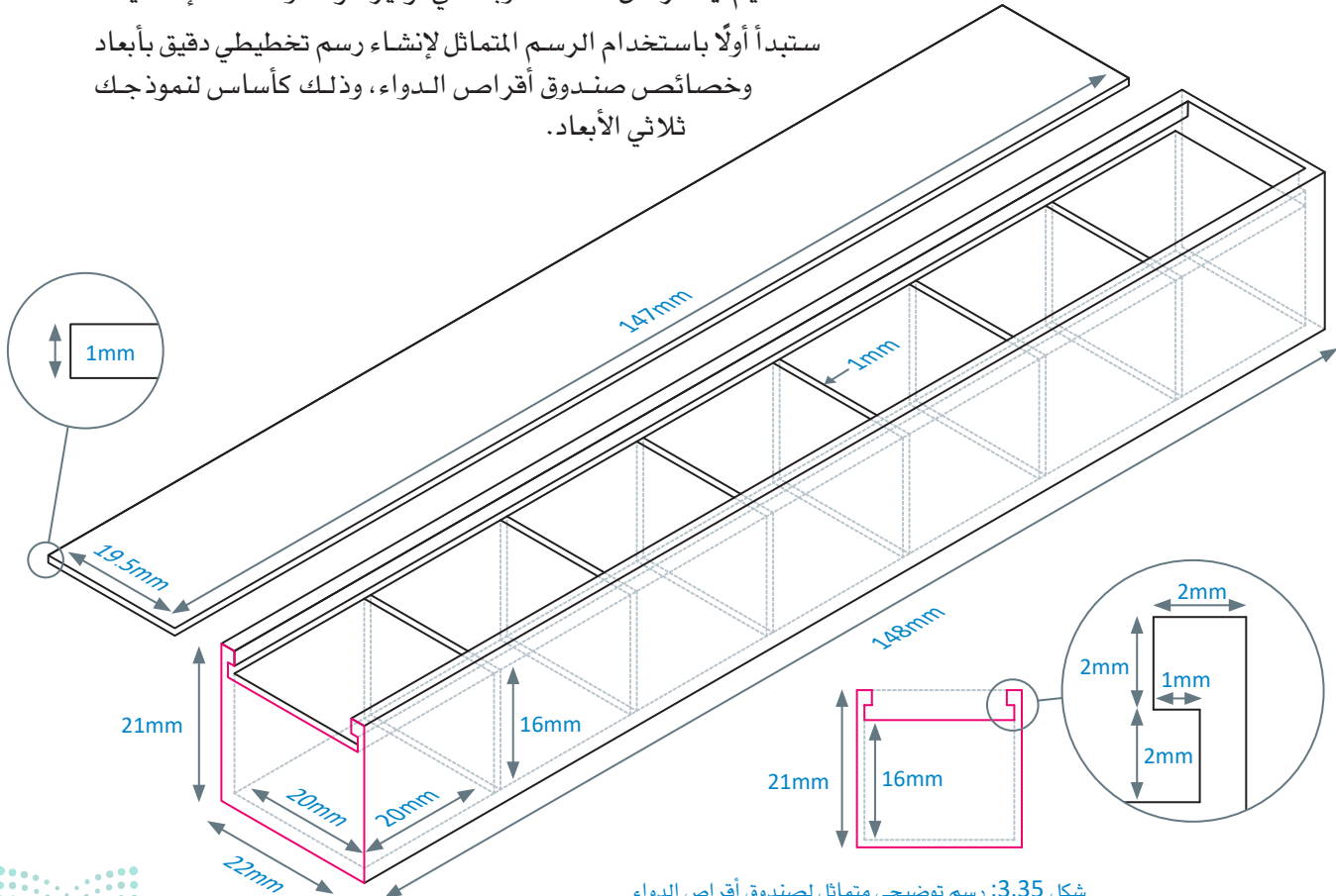
شكل 3.35: رسم توضيحي متماثل لصندوق أقراص الدواء
