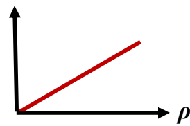
الضغط وكثافة السائل
