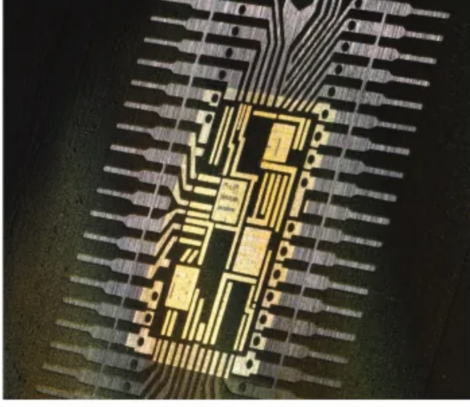
الشكل 18 هذه الرفاقة الدقيقة توصل الكهرباء عند درجات الحرارة المرتفعة باستخدام شبه موصل.
