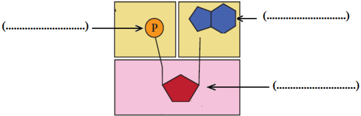
تركيب النيوكليوتيدة
