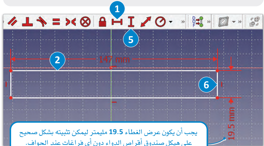
شكل 3.60: تقييد المسافة الأفقية والرأسية
