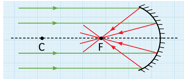
الشكل (2) البؤرة في المراة المقعرة
