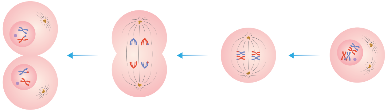
المرحلة التمهيديّة الأولى المرحلة الاستوائيّة الأولى المرحلة الانفصاليّة الأولى المرحلة النهائيّة الأولى الشكل (5 أ) الانقسام الميوزي الأوّل
