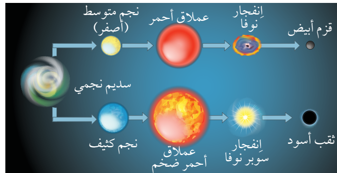
الشكل (8) دورة حياة النجوم
