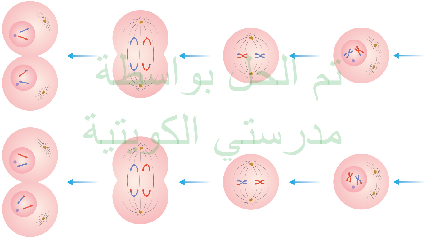
المرحلة التمهيديّة الثانية المرحلة الاستوائيّة الثانية المرحلة الانفصاليّة الثانية المرحلة النهائيّة الثانية الشكل (5 ب) الانقسام الميوزي الثاني
