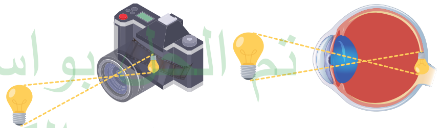
الشكل (31) عمل العين والكاميرا
