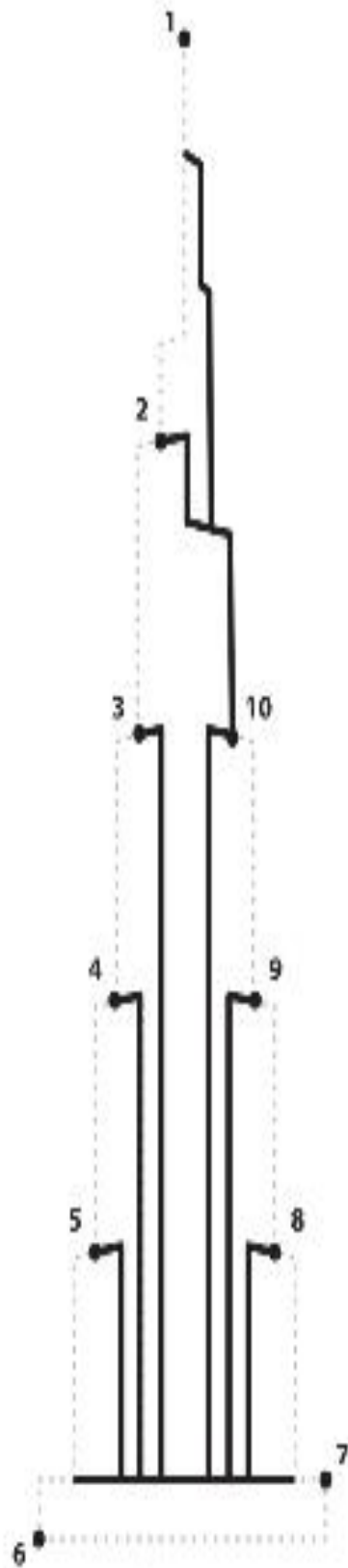
بُرْجُ خَلِيفَةٍ
